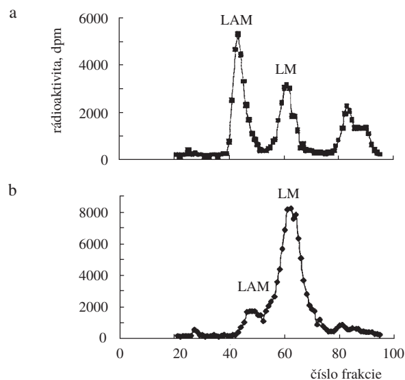
Obr. 2. Gélová filtrácia deacylovaných lipoarabinomananových frakcií na kolóne (118×1 cm) s náplňou Bio-Gel P 100. Na kolónu sa nanieslo 120 000 dpm vzorky po hydrolýze v 0,1 M-NaOH (2 hod, 37 °C). Zbierané frakcie mali objem 1,2 ml; a – LM/LAM frakcia kontrolnej kultúry; b – LM/LAM frakcia kultúry inhibovanej 100 µg.m -1 A11
