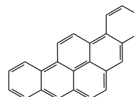
Dibenzo[a,i]pyren
