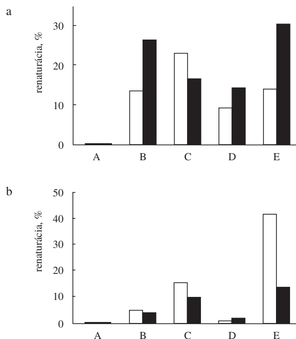
Obr. 1. a) Závislosť renaturácie MDH v prítomnosti BSA, OAA a glycerolu, (denaturácia 4,5 mol.l -1 močovinou), b) závislosť renaturácie MDH v prítomnosti BSA, OAA a glycerolu (denaturácia 1,2 mol.l -1 guanidínhydrochloridom); ■ 20-násobné riedenie denaturovanej MDH, □ 50-násobné riedenie denaturovanej MDH; renaturácia: A – 20 mmol.l -1 Tris-HCl pH 8,0, 50 mmol.l -1 2-ME, B – 0,5 mmol.l -1 OAA, 6 μmol.l -1 BSA, 25 % glycerol v roztoku A, C – 0,5 mmol.l -1 OAA, 6 μmol.l -1 BSA v roztoku A, D – 0,5 mmol.l -1 OAA, 25 % glycerol v roztoku A, E – 6 μmol.l -1 BSA, 25 % glycerol v roztoku A
